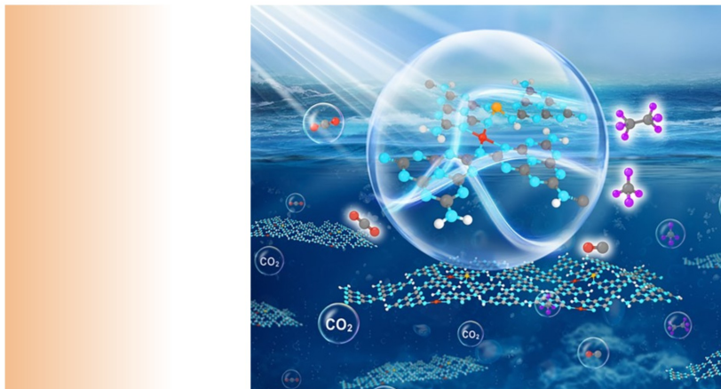
CO 2 还原的示意图
